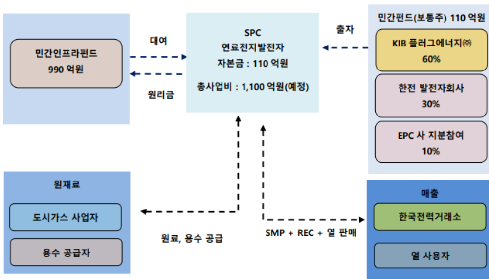
그림 10. 연료전지 발전소 사업구조 예시
